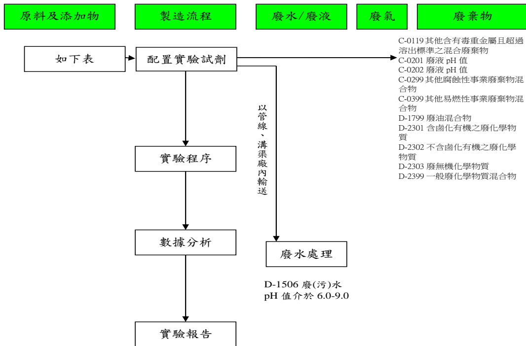
製程流程圖 (850001 化學(農化)實驗作業程序)
